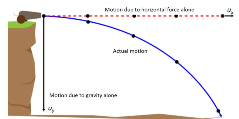
Figur 2.2: Prosjektilbevegelse
